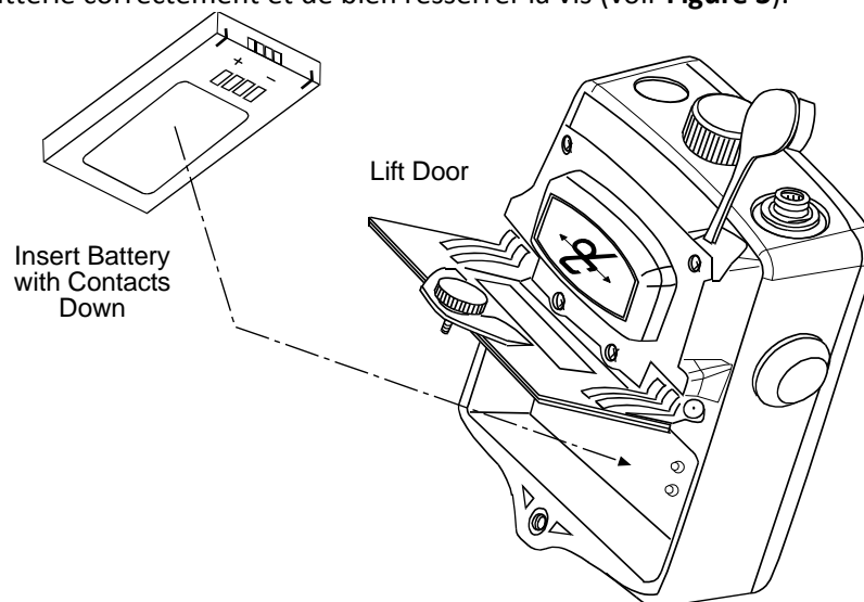
Figure 3 : Insertion/Retrait de la batterie
