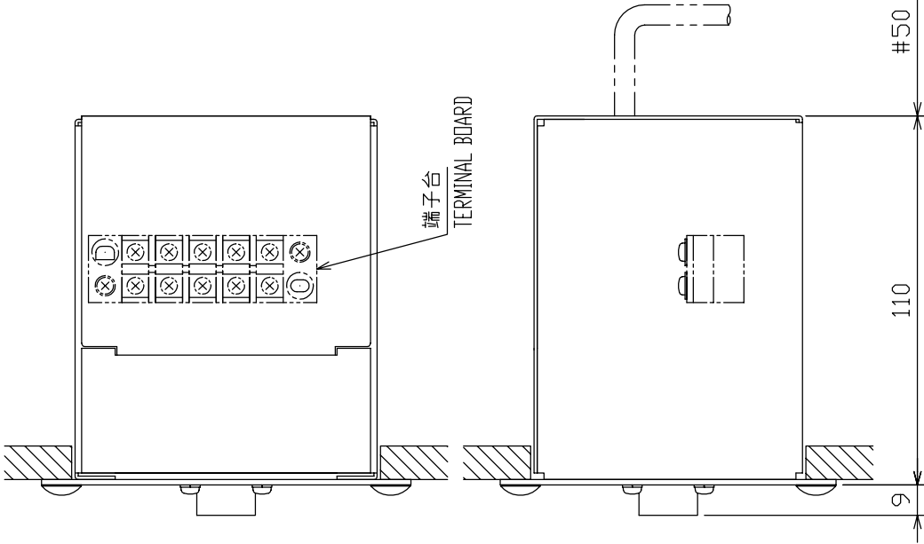
取付寸法図（参考図） CUTOUT DIMENSIONS
