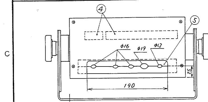
背面図 REAR VIEW
