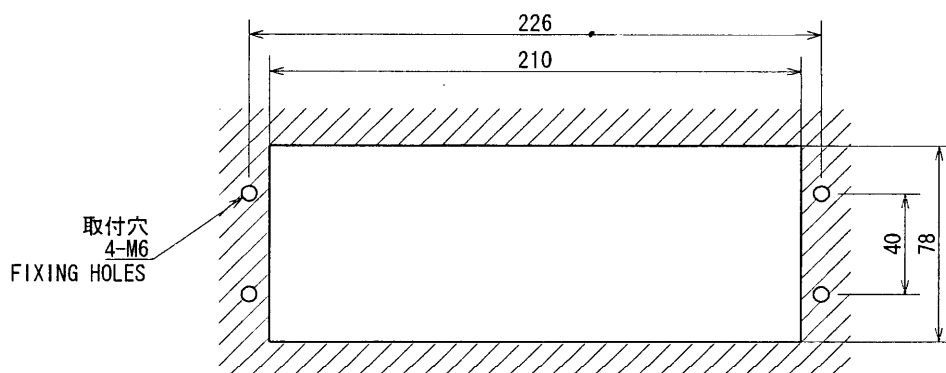
取付穴寸法 CUTOUT DIMENSIONS
