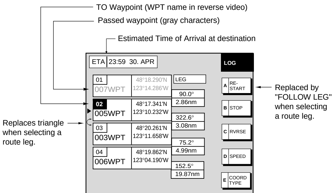
Log display
