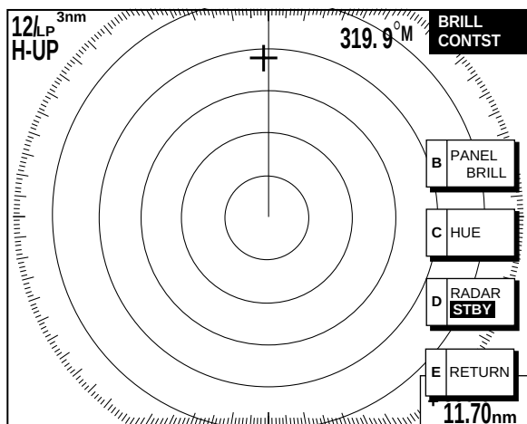
Radar Display
