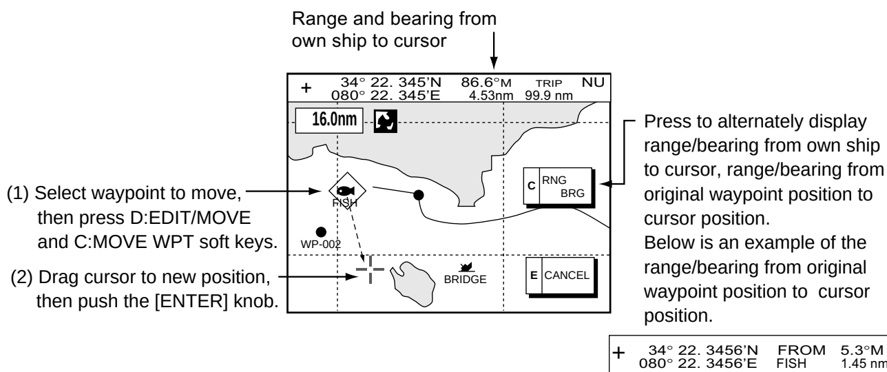
Plotter display
